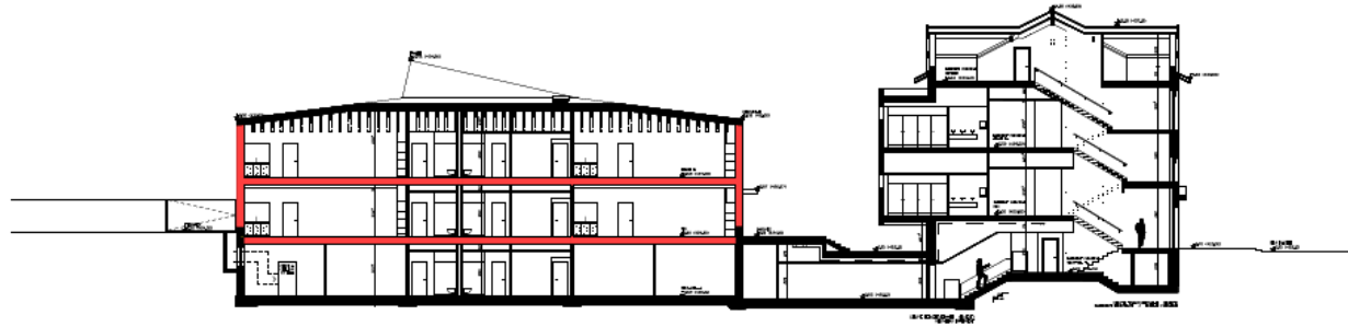
Coupe D-D
