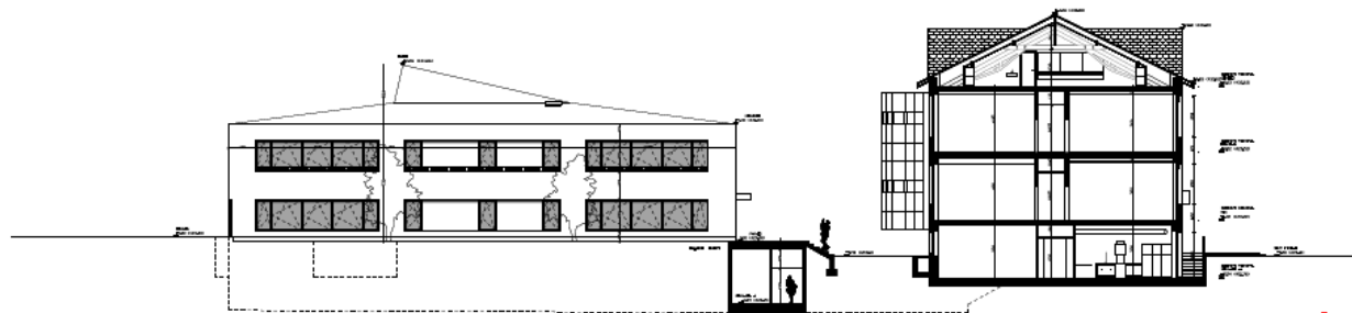
Façade Ouest
